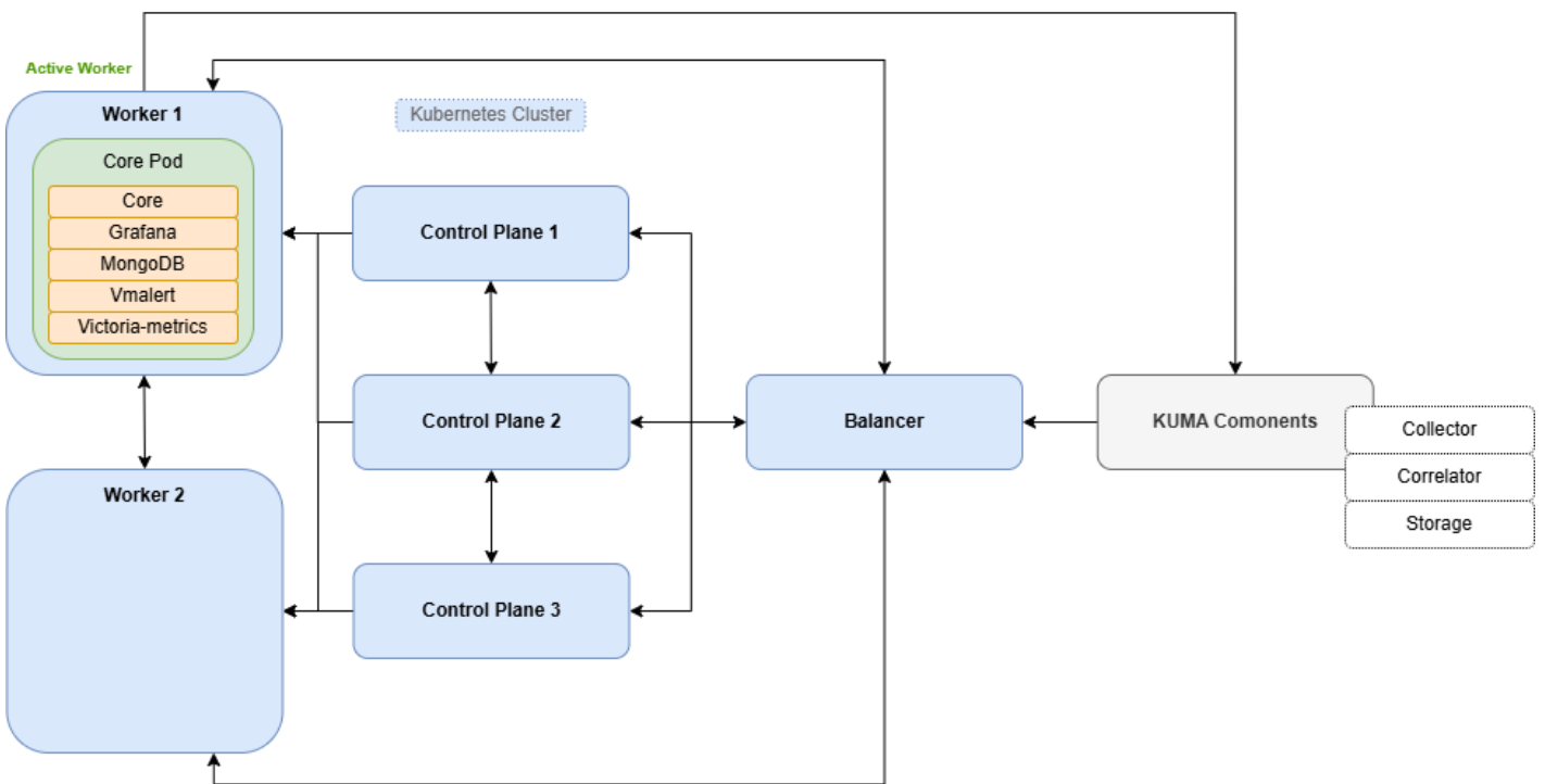
Схема работы в случае отказа одного из воркеров ядра
